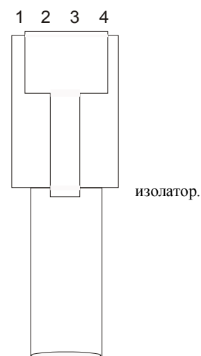
СЪЕДИНИТЕЛ RJ11 Разположение на изводите
